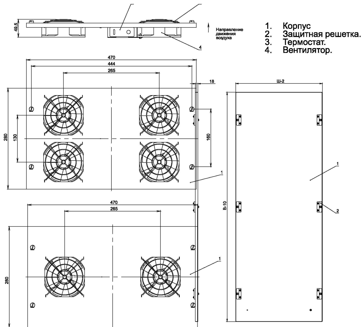
Схема БВ-2-Т-7035 и БВ-4-Т-7035
